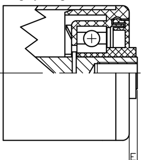
Подшипниковый корпус серии LB
